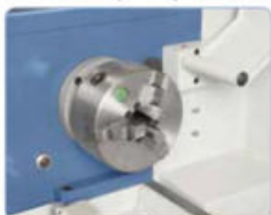
Ventajas del plato Bernardo DK11-160: Disponibles garras blandas, superiores blandas y duras.
